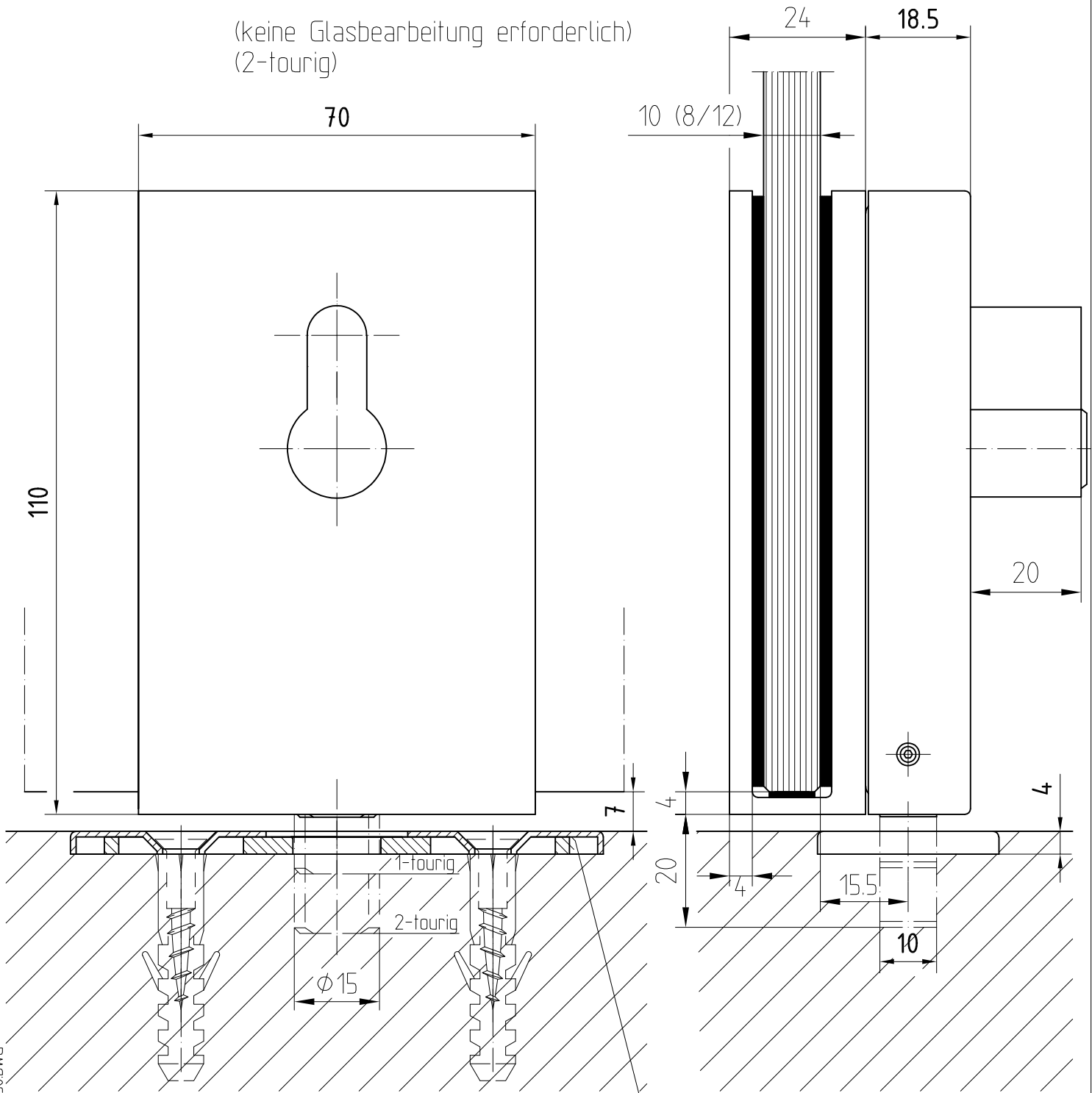
Schließblech Art. Nr. 05.190
