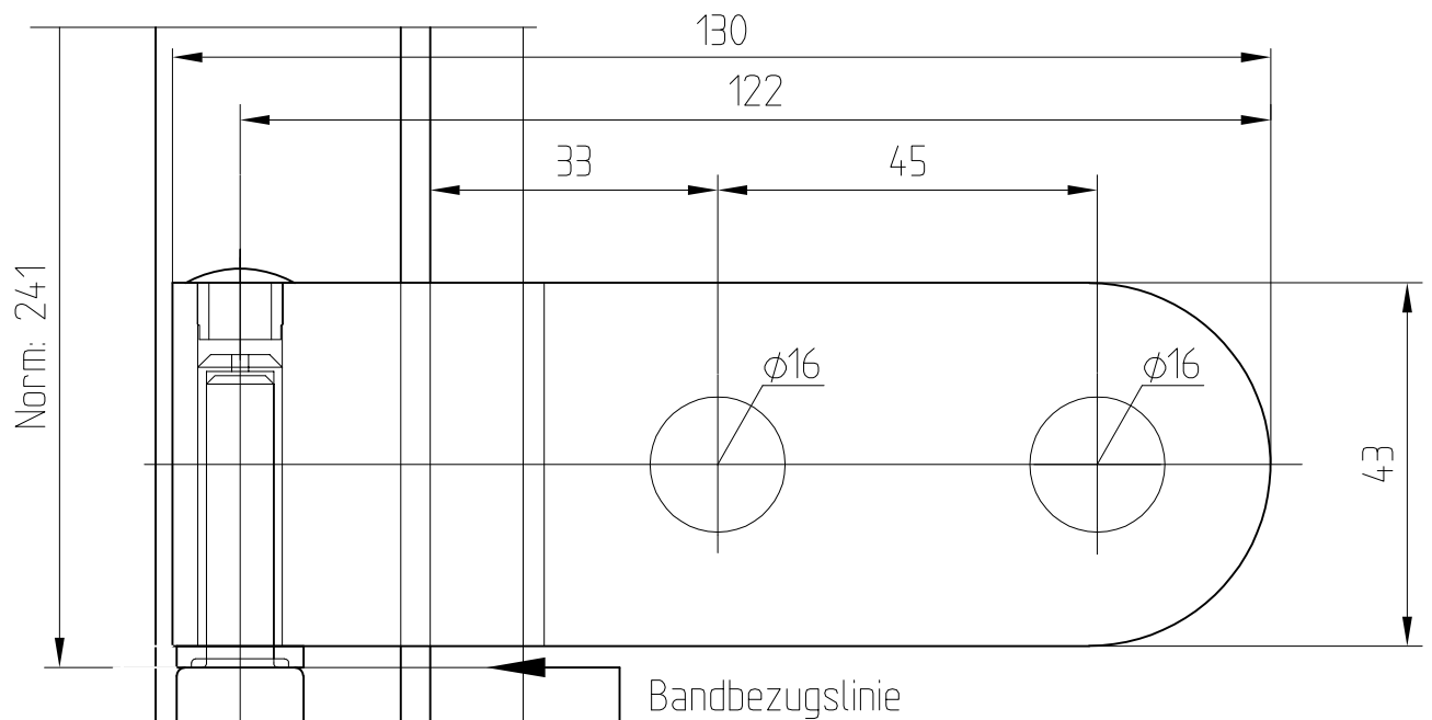
Abb. 24mm Falztiefe
