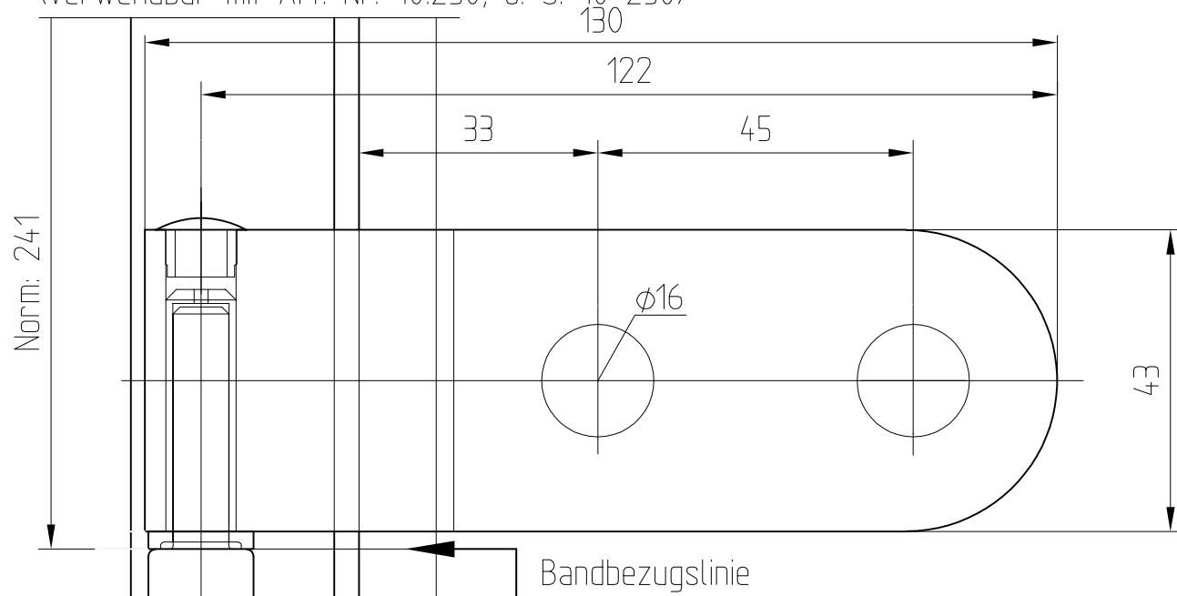
Abb. 40mm Falztiefe
