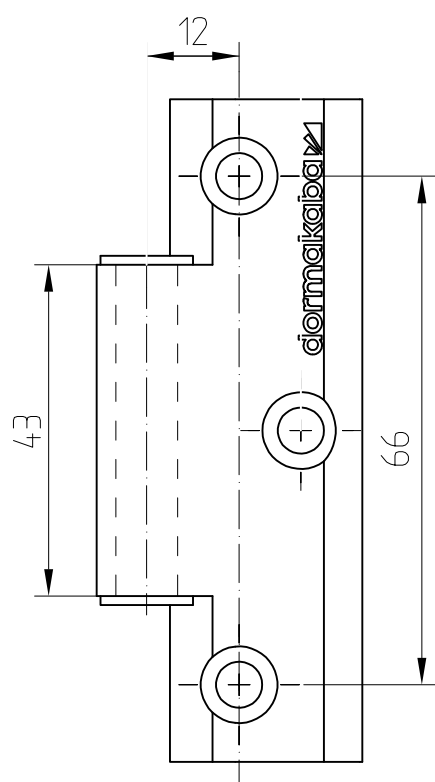
Ansicht Rahmenteil
