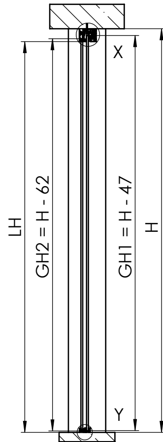
A-A (1 : 20)
