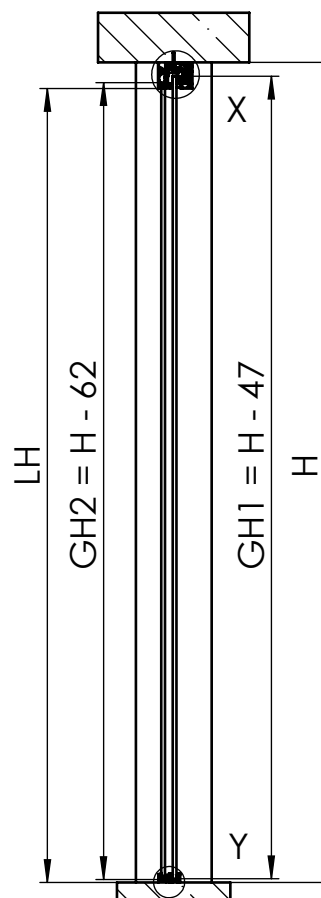
A-A (1 : 20)
