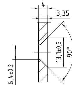
Detail Befestigungsbohrung Laufschiene
