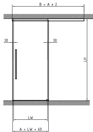
Einzelflügel an Decke
