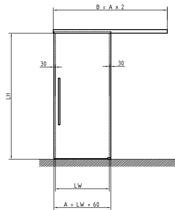
Einzelflügel an Wand
