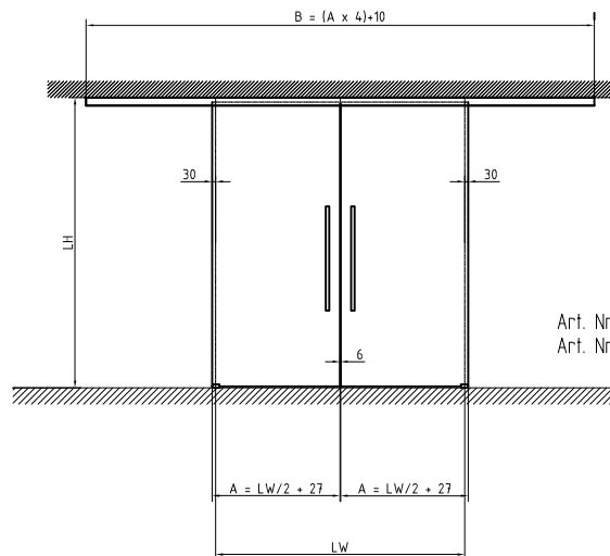
Doppelflügel an Decke
