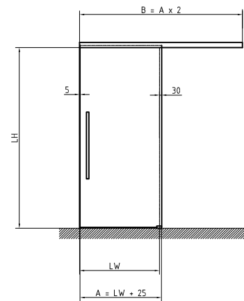
Einzelflügel vor Wand laufend
