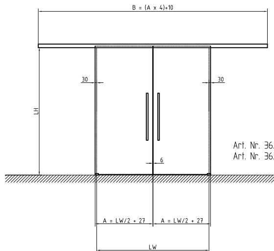
Doppelflügel an Wand
